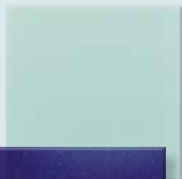
Ätzeffekt
